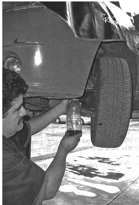
Al presionar el pedal se abre el tornillo purgador
