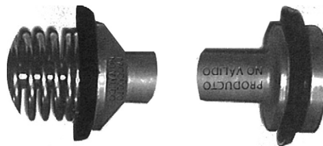
Gomas primaria y secundaria hinchadas
