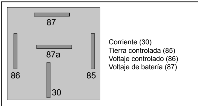
Relevador
