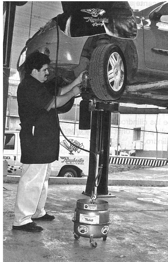
Purgado con tanque de purga a presión
