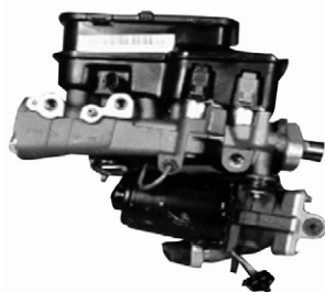
Frenos ABS tipo integral o cerrado
