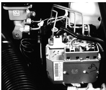
Frenos ABS tipo no integral o abierto
