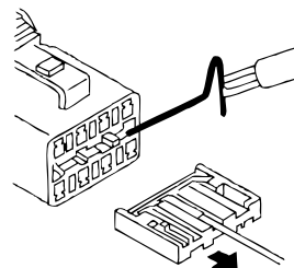
Seguro conector
